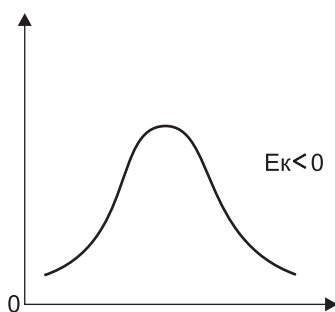
Рис. 7.6. Плосровершинное распределение
